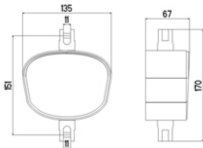
ABMESSUNGEN (mm)
